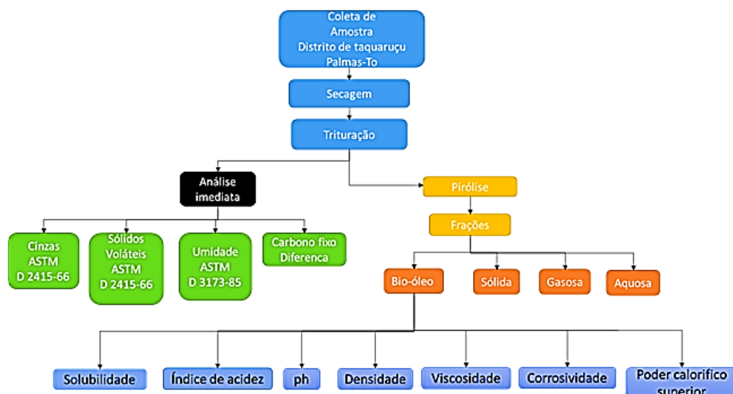
Figura 1. Fluxograma do preparo da biomassa de babaçu e produção e caracterização do bio-óleo (Os autores, 2020)
