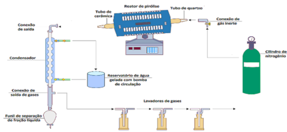
Figura 4. Desenho esquemático da unidade de pirólise em escala laboratorial do LEDBIO – UFT (Fonte: Correia, 2013).
