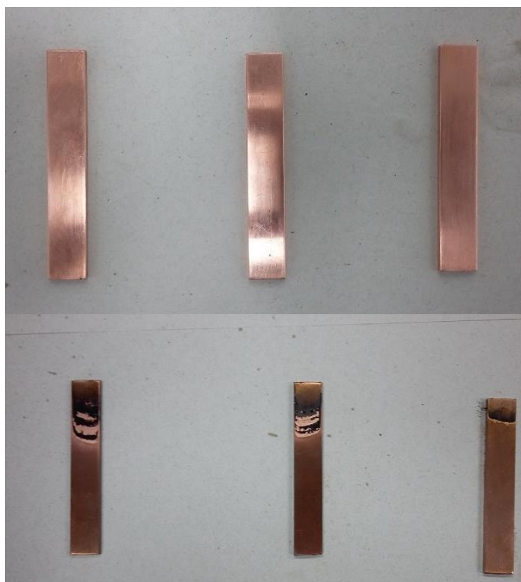
Figura 5. Lâminas de cobre após o ensaio de corrosividade com as amostras de bio-óleo de babaçu (Os autores, 2020)
