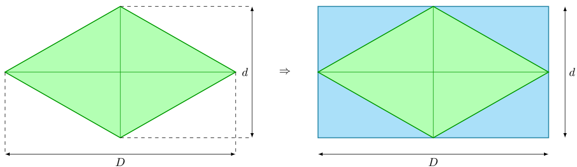
Figura 12 – Losango
