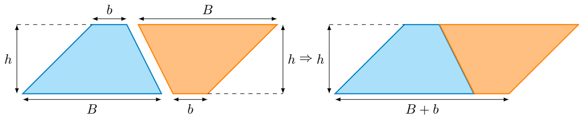
Figura 13 – Trapézio
