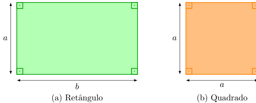
Figura 10 – Quadriláteros Retangulares
