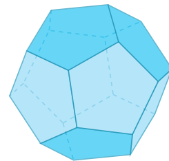
Dodecaedro
