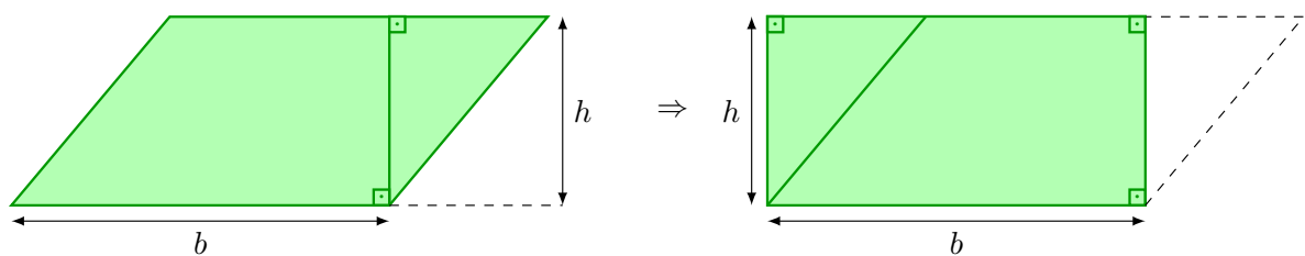
Figura 11 – Paralelogramo
